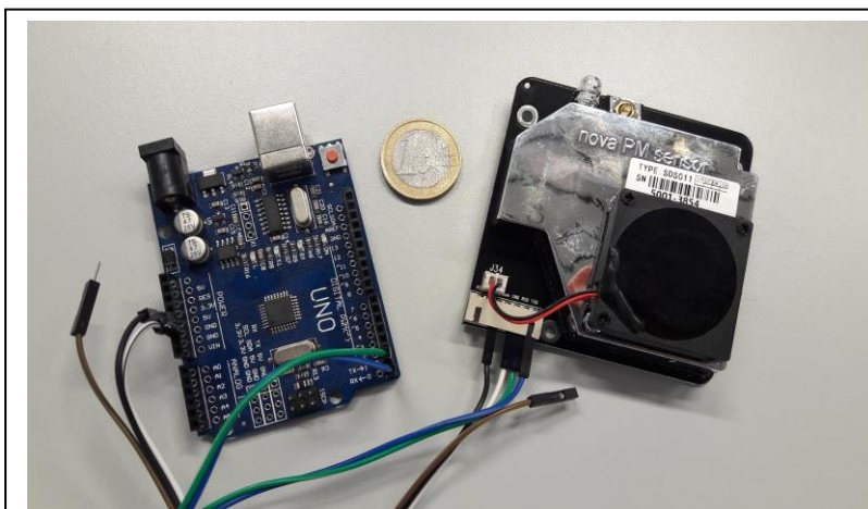
Foto: Sensor SDS011
