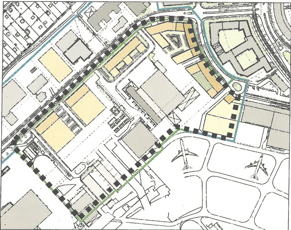
Abbildung 1: Ausschnitt städtebaulicher Masterplan (Verfasser: Westphal Architekten BDA, Bremen)
